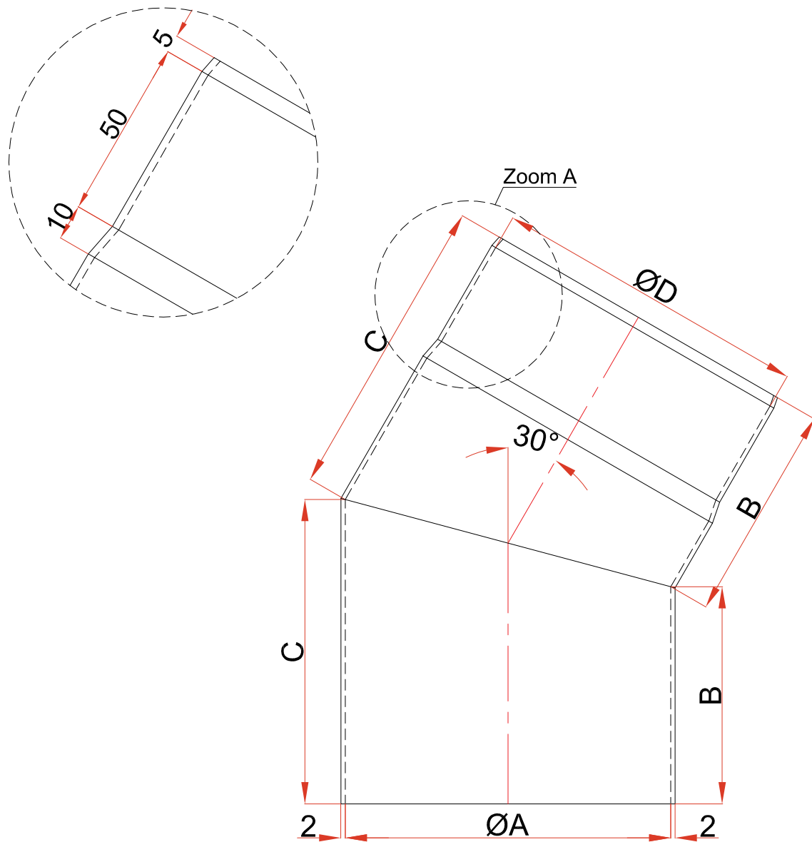
Dimensions (en mm) / afmetingen (mm)
