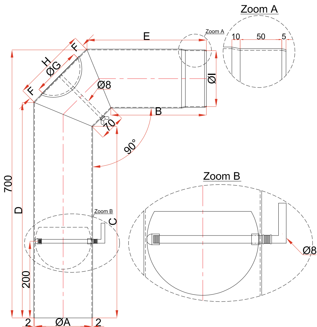
Dimensions (en mm) / afmetingen (mm)
