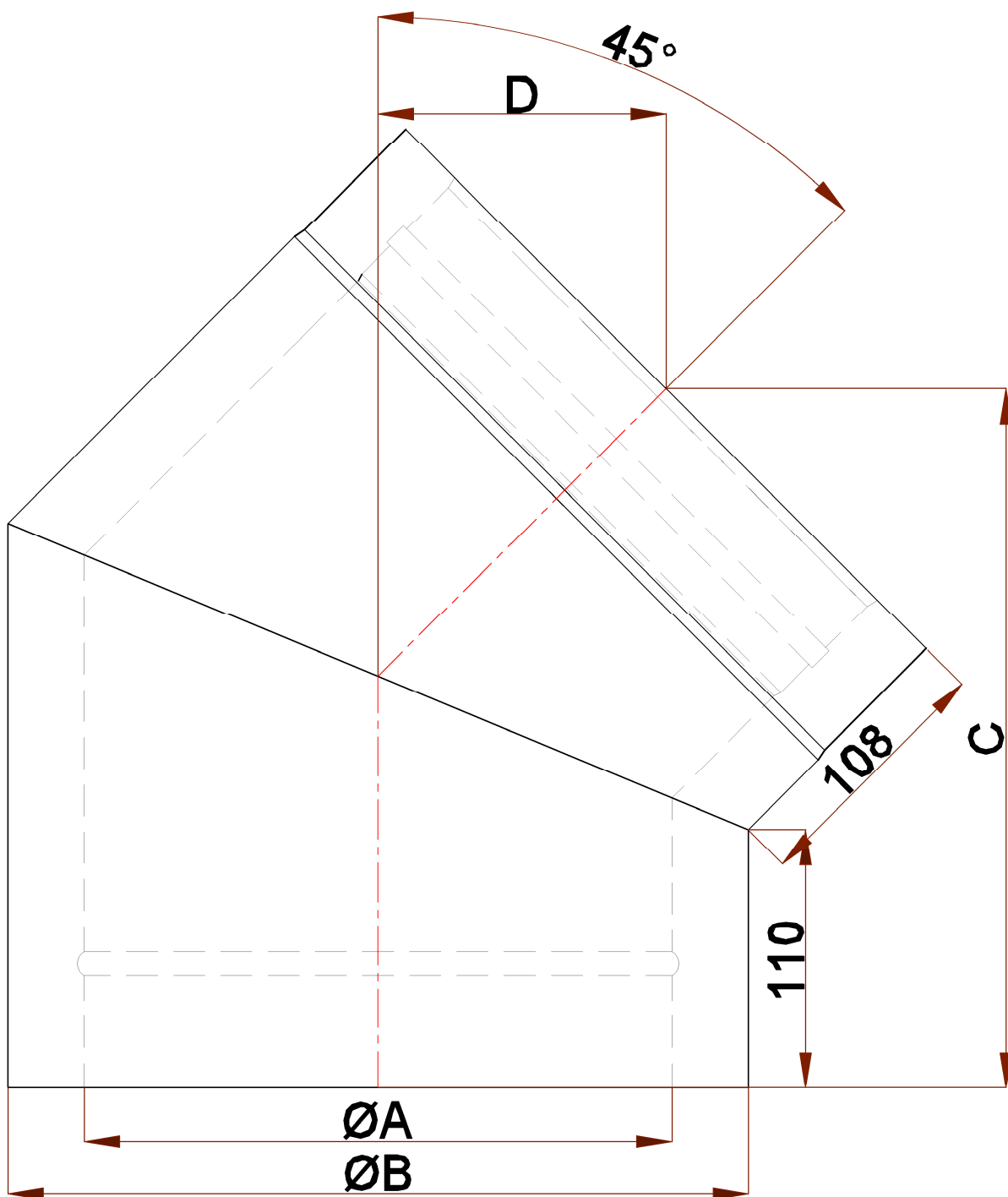
Dimensions (en mm) / afmetingen (mm)
