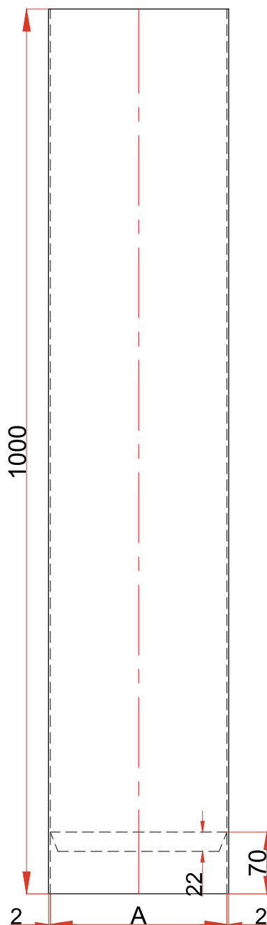
Dimensions (en mm) / afmetingen (mm)
