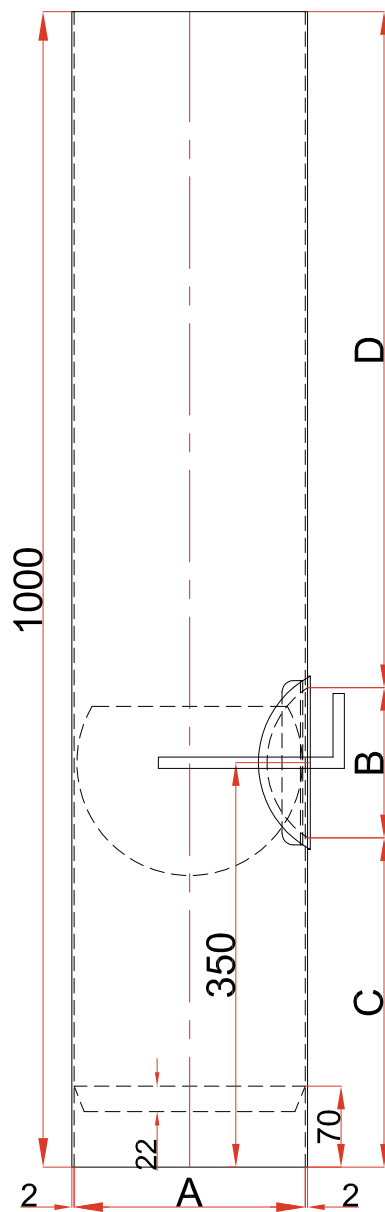
Dimensions (en mm) / afmetingen (mm)
