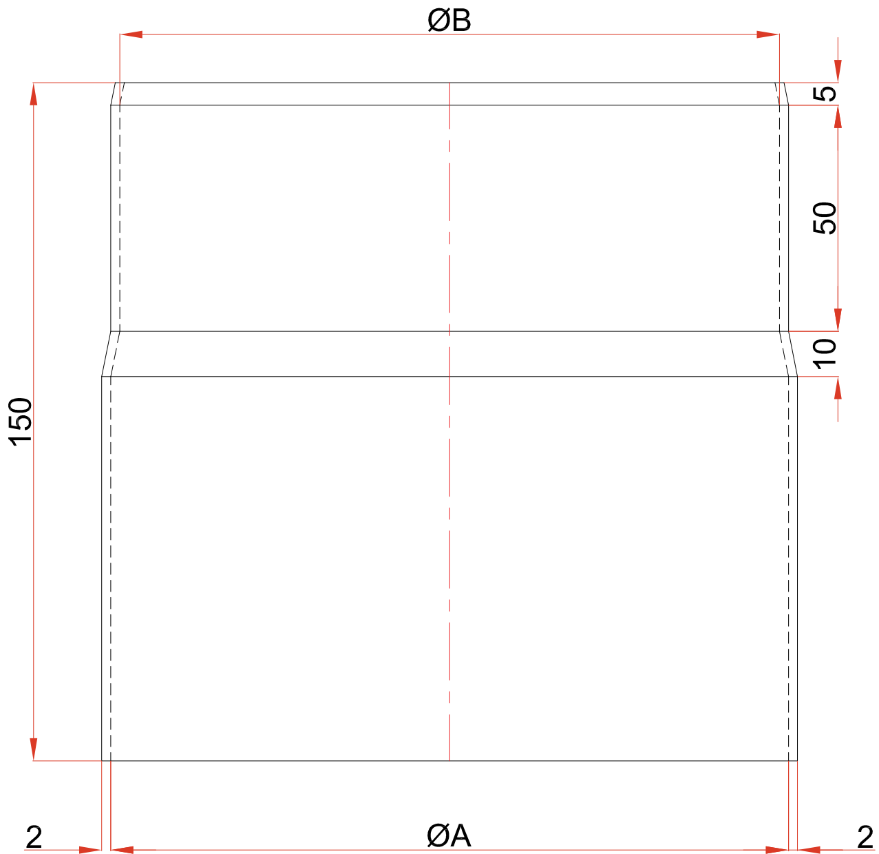
Dimensions (en mm) / afmetingen (mm)
