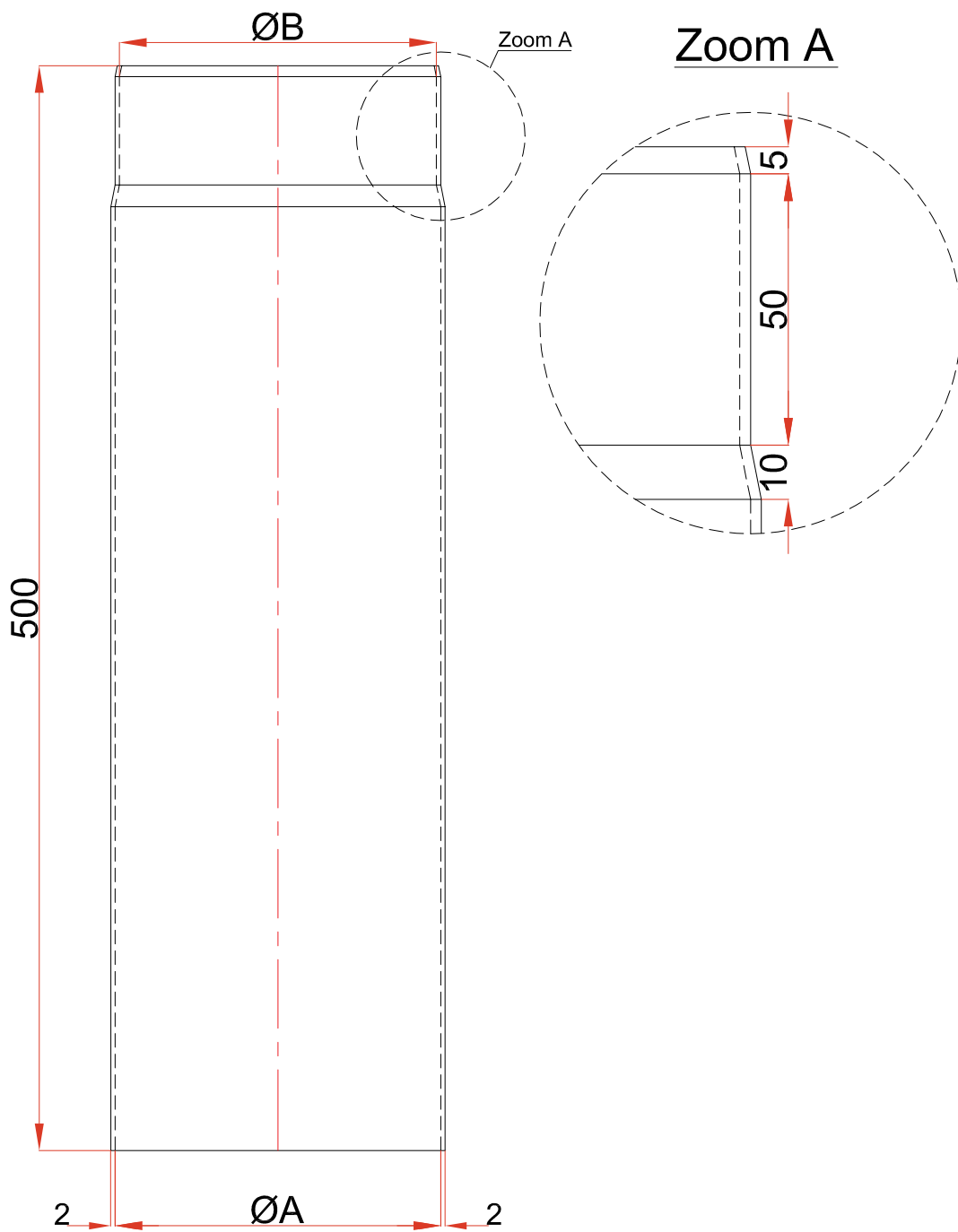
Dimensions (en mm) / afmetingen (mm)
