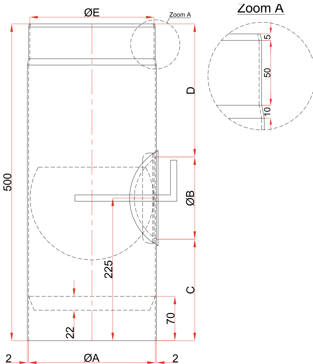
Dimensions (en mm) / afmetingen (mm)
