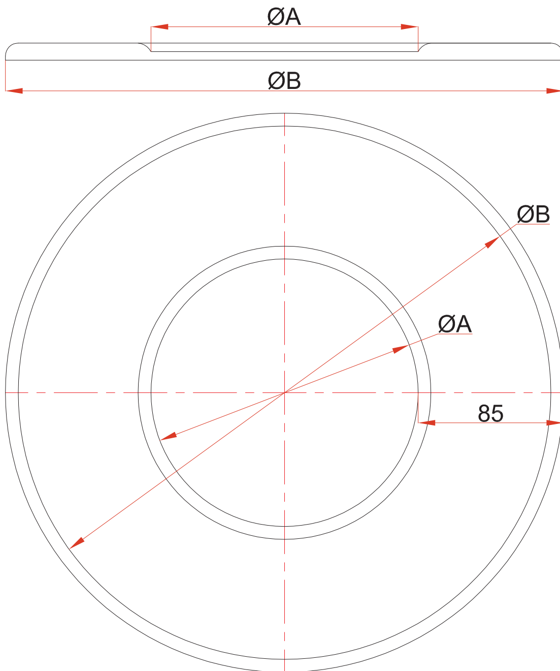
Dimensions (en mm) / afmetingen (mm)
