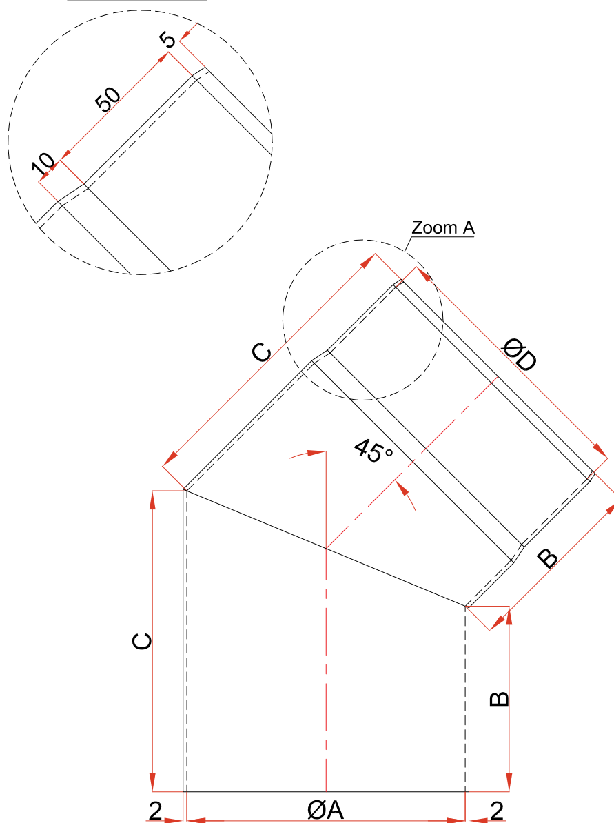
Dimensions (en mm) / afmetingen (mm)
